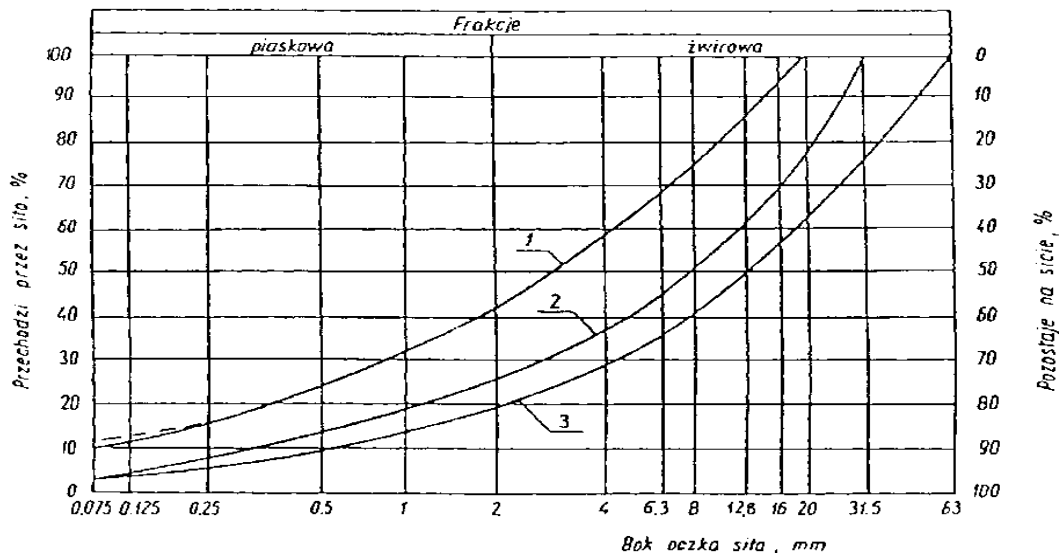
Rysunek 1. Pole dobrego uziarnienia kruszyw przeznaczonych na podbudowy (fundamenty) wykonywane metodą stabilizacji mechanicznej
